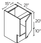
1 DOOR 15" | V15ADA(L/R)
