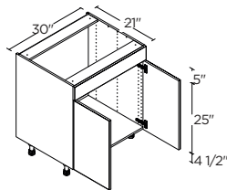
2 DOORS 30" | VS30
