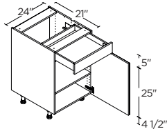
1 DOOR / 1 DRAWER 24" | V24(L/R)
