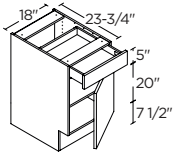
1 DOOR / 1 DRAWER 18" | B18ADA
