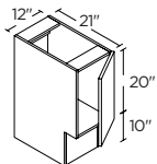
1 DOOR 12" | V12ADA(L/R)
