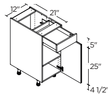
1 DOOR / 1 DRAWER 12" | V12(L/R)
