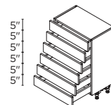
6 DRAWERS 15" | B6D1514 18" | B6D1814 24" | B6D2414
