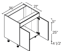
2 DOORS 36" | VS36
