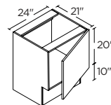
1 DOOR 24" | V24ADA(L/R)
