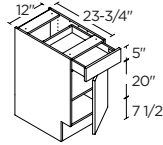
1 DOOR / 1 DRAWER 12" | B12ADA
