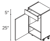
1 DOOR / 1 DRAWER 15" | B1514(L/R) 18" | B1814(L/R) 24" | B2414(L/R)
