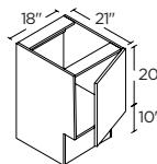
1 DOOR 18" | V18ADA(L/R)
