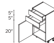
1 DOOR / 2 DRAWERS 15" | B1514B(L/R) 18" | B1814B(L/R) 24" | B2414B(L/R)
