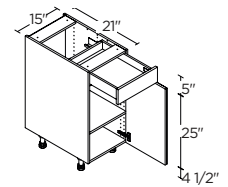
1 DOOR / 1 DRAWER 15" | V15(L/R)
